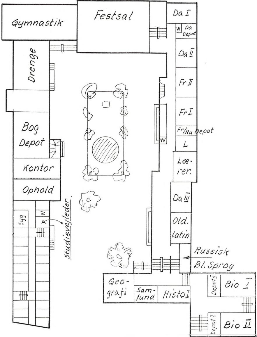
Stueplan
