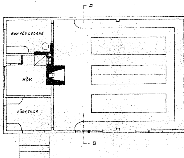
LÄROVERKETS SPORTSTUGA (PLANRITNING).
