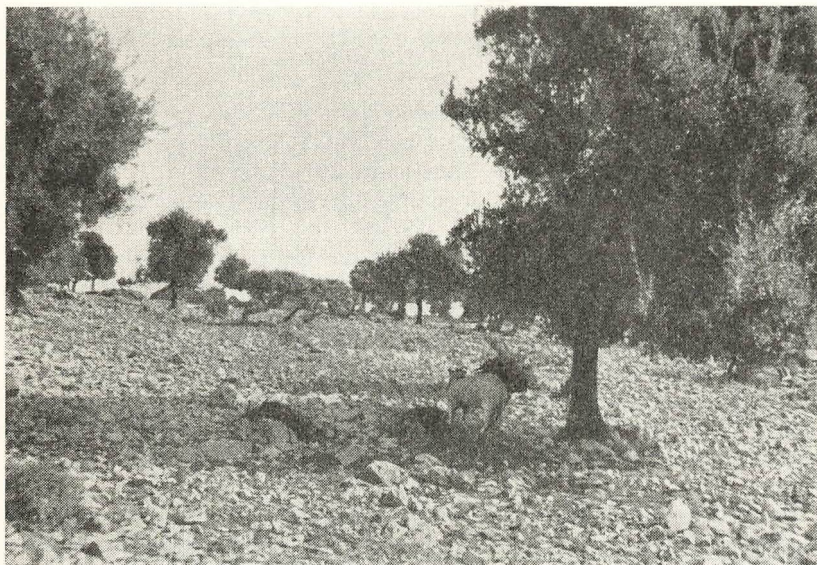
På den nordlige ende af Kamenjak breder sig en åben skov, Kalifront, af stene og træformede enebær. Færene søger skygge i middagsheden.
