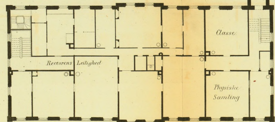
2 den Etage
