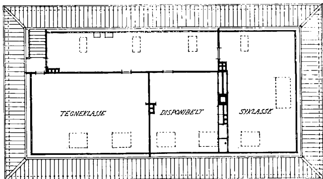
PLAN AF TAGE TAGE
