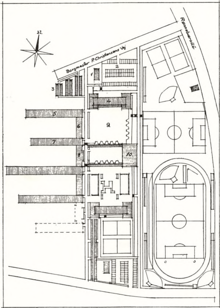
Grundplan over skolekomplekset ved Rønnebærrallé. Gymnasiet: 1. Pedelbolig. – 2. Parkeringsplads for biler. – 3. Cykel-parkering. – 4. Gymnastiksale. – Særklassefløj. – 6. Lærerværelser. – 7. Normalklassefløj. – 8. Kontorer. – 9. »Legeplads«. – 10. Festsal og kantine.
