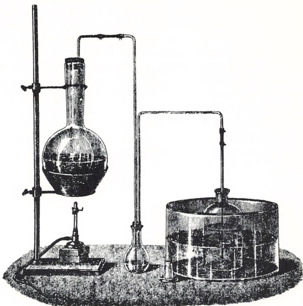
Fremstilling af salmiakspiritus (anno 1900).
