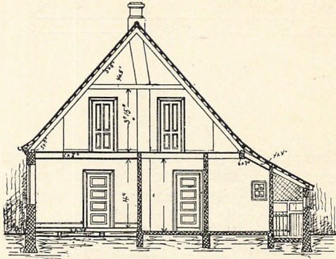
Snit a. b.
