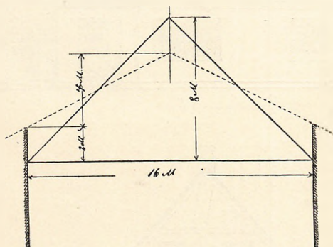
Rids af Tagværk.
