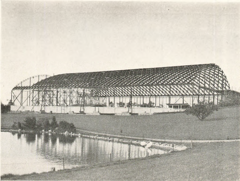
Idrætshallens Staalskelet.
