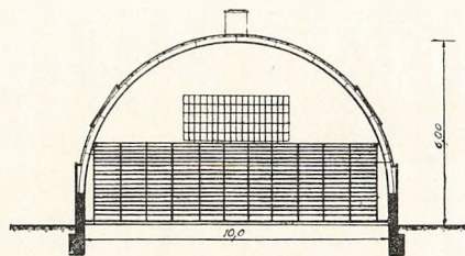
Tværsnit i Sal
