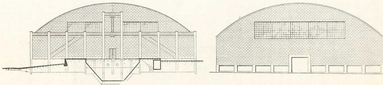
Idrætshallens Gavle.
