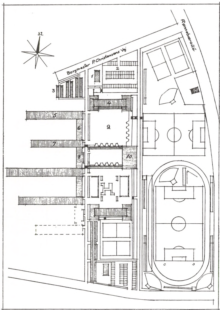
Grundplan over skolekomplekset ved Rønnebæralle. Gymnasiet: 1. Pedelbolig. — 2. Parkeringsplads for biler. — 3. Cykelpar- kering — 4. Gymnastiksale. — 5. Særklassefløj. — 6. Lærervæ- relser. — 7. Normalklassefløj. — 8. Kontorer. — 9. »Legeplads«. — 10. Festsal og kantine.
