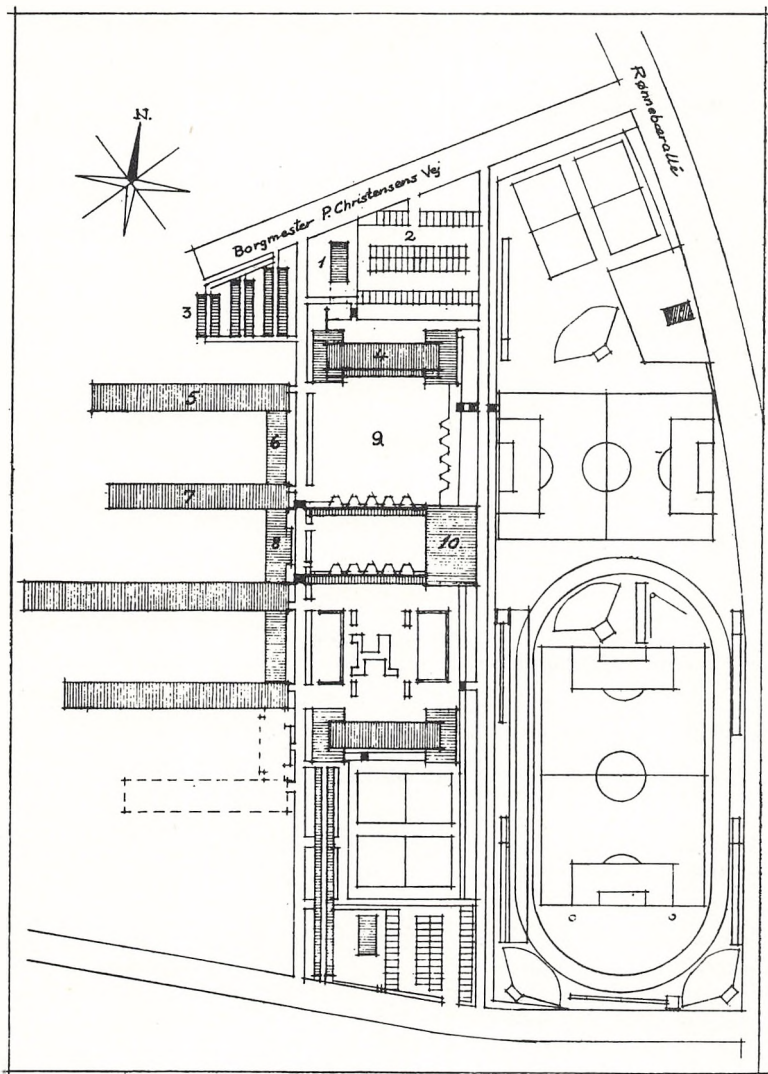
Grundplan over skolekomplekset ved Rønnebæralle. Gymnasiet: 1. Pedelbolig. — 2. Parkeringsplads for biler. — 3. Cykelpar- kerer — 4. Gymnastiksale. — 5. Særklassefløj. — 6. Lærervæ- relser. — 7. Normalklassefløj. — 8. Kontorer. — 9. »Legeplads«. — 10. Festsal og kantine.
