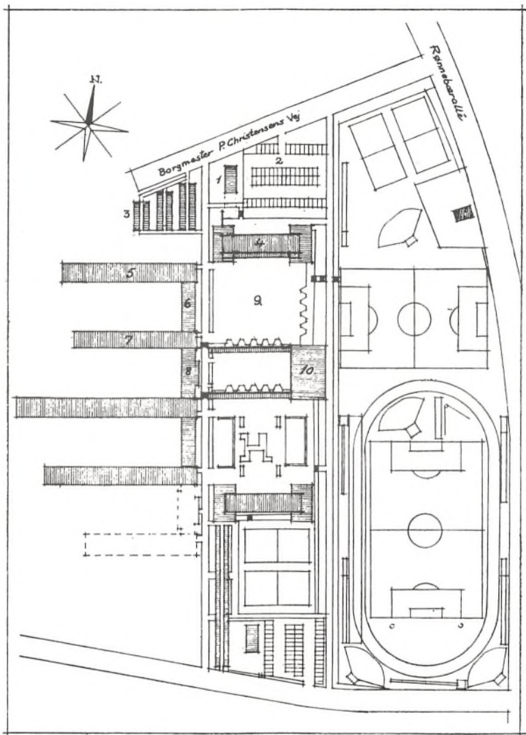
Grundplan over skolekomplekset ved Rønnebærallé. Gymnasiet: 1. Pedelbolig. — 2. Parkeringsplads for biler. — 3. Cykelpar- kering — 4. Gymnastiksale. — 5. Særklassefløj. — 6. Lærervæ- relser. — 7. Normalklassefløj. — 8. Kontorer. — 9. »Legeplads«. — 10. Festsal og kantine.
