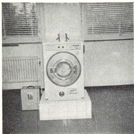
Den helautomatiske vaskemaskine med hulkortsystemet. Ved siden af ses en transportabel el-måler.
