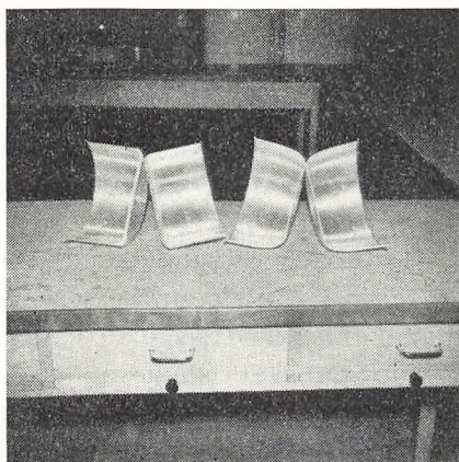
To gennemskårne al-gryder, den ene tyndbundet, den anden tykbundet og planslebet. Med disse kan man rigtigt demonstrere forskellen.
