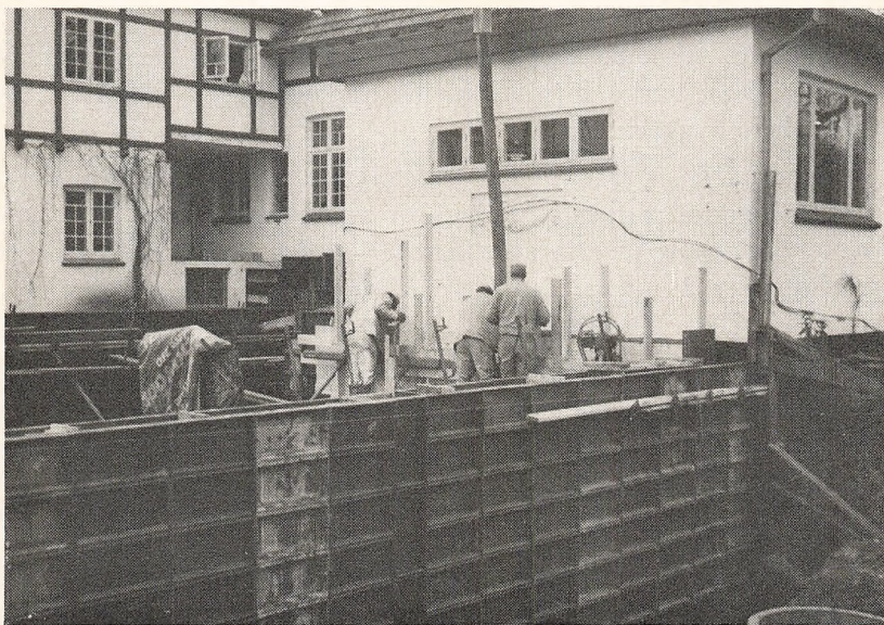
Støbning af fundament – på 1 dag.
