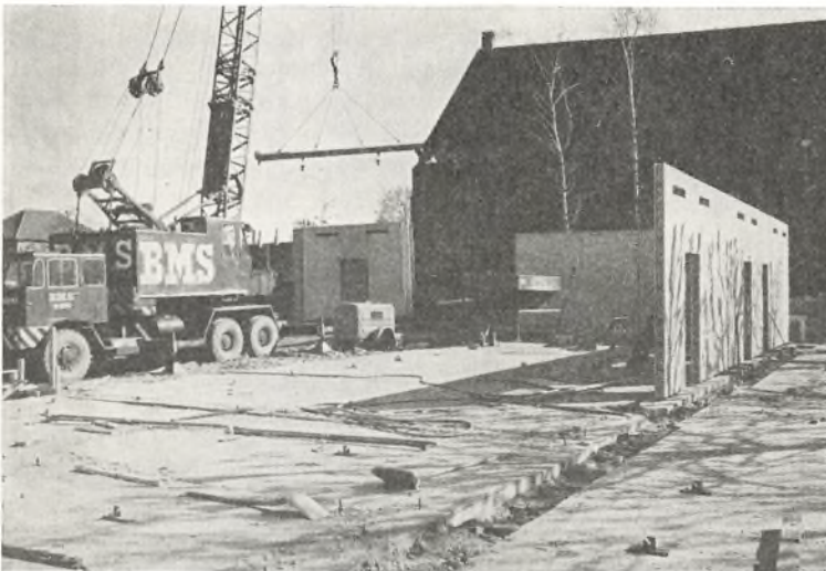
Tilbygning til Skolen i Lundegade. De første elementer bringes på plads.
