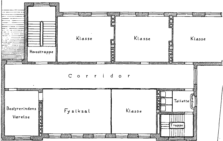
Plan af 1 ste Sal
