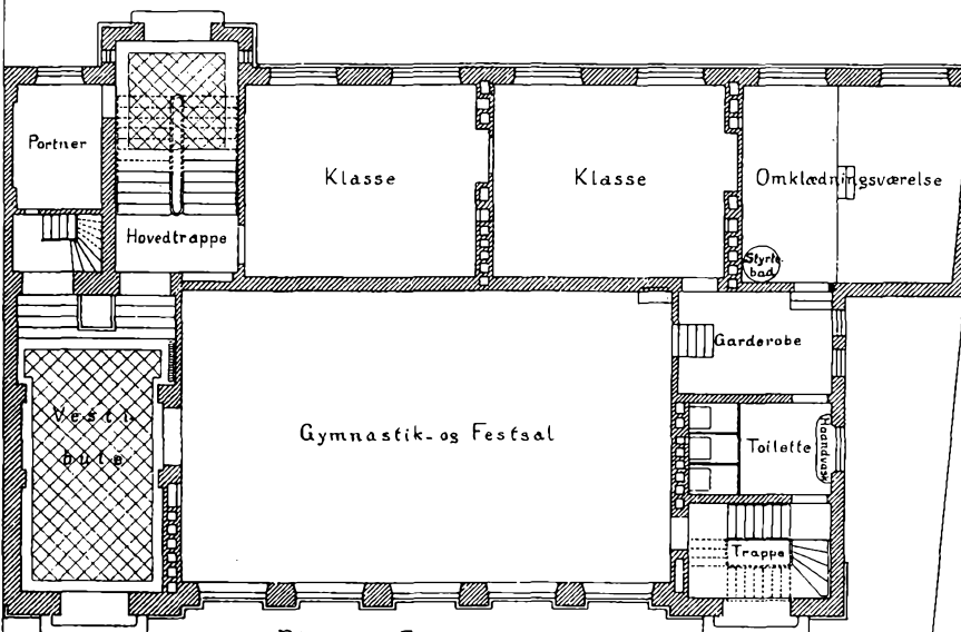
Plan af Stueetagen
