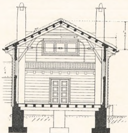
TVÆRSNIT
