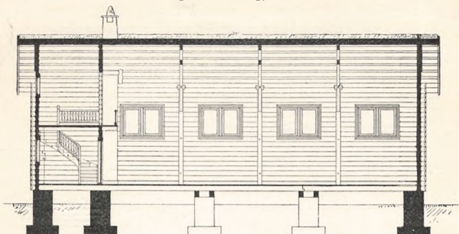
LÆNGDESIT
