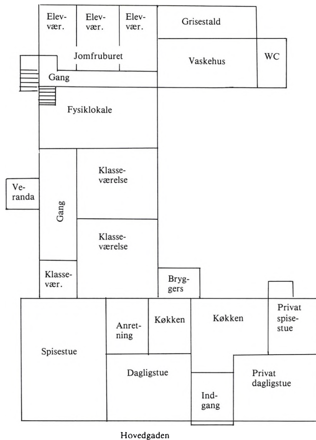
Plan over Høng Gymnasium fra 1930'erne. Tegnet efter Karsten Munks beskrivelse.
