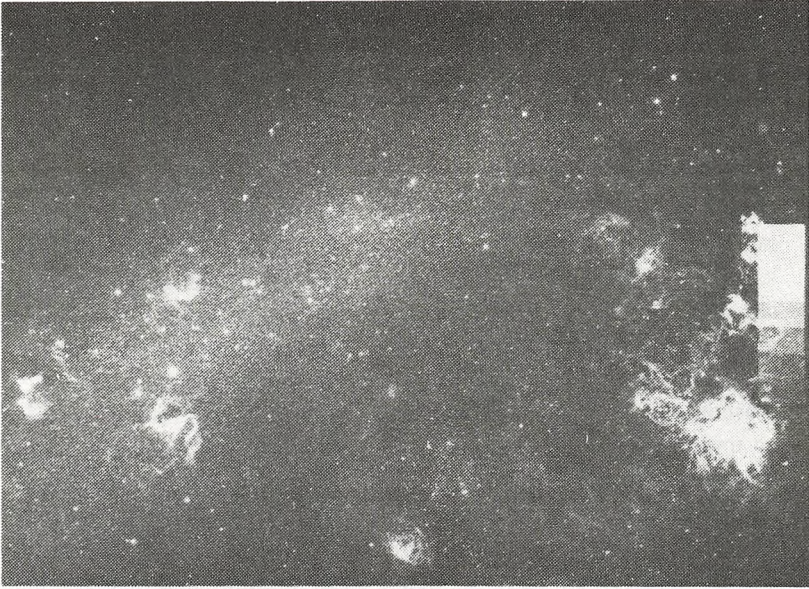
Den Store Magellanske Sky.
