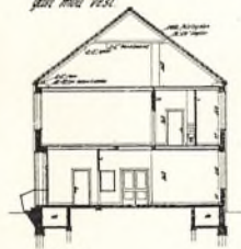
snit b-b
