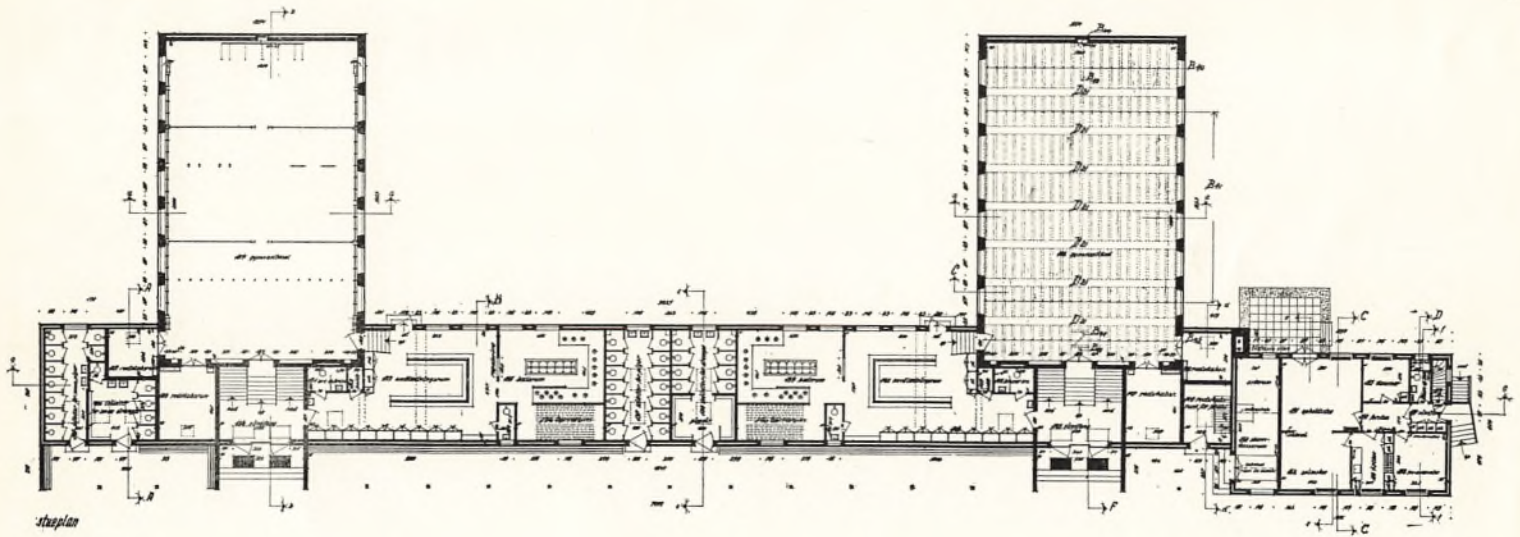
stueplan
