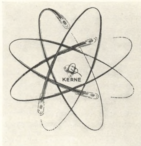
Den moderne atomfysik har skaffet os sikker indsigt i opbygningen af stoffets mindste dele: de udelelige atomer. På grundlag af de resultater, som to af atomforskningens største navne, englænderen Rutherford og danskeren Niels Bohr er kommet til, har man for at anskueliggøre atomet konstrueret en såkaldt atommodel, der kan lignedes ved et miniatyresolsystem med atomkernen på solens plads og elektronerne kredsende som planeter udenom.
