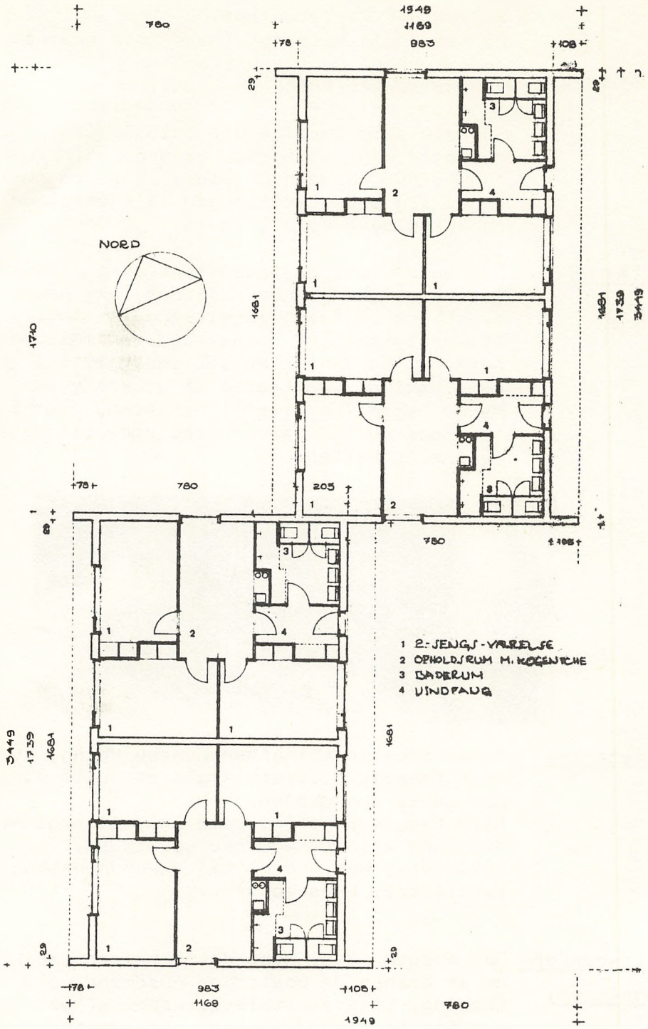
STUEPLAN
