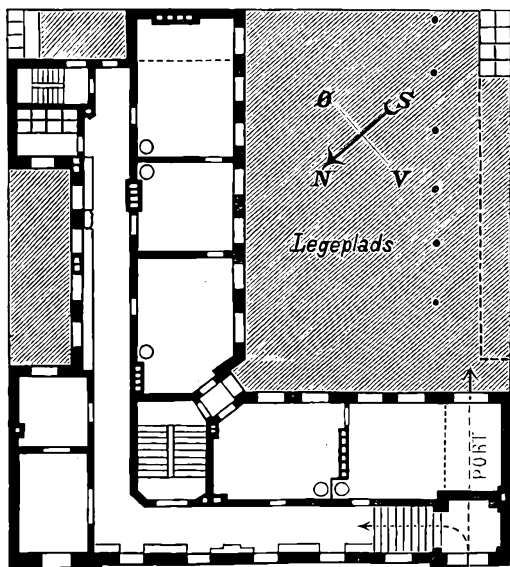
Grundrids af Stuen.
