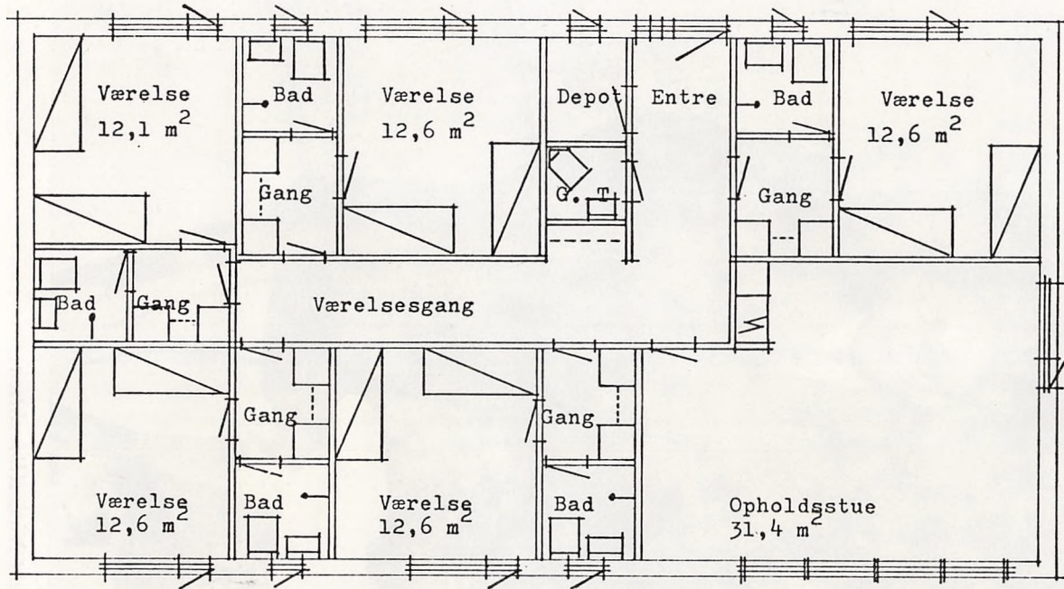
Grundplan af ét af de seks typehuse, der skal være bolig for 10 elever.
