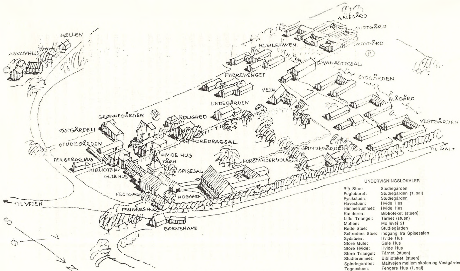
ASKOV HØJSKOLE · OVERSIGTSPLAN.
