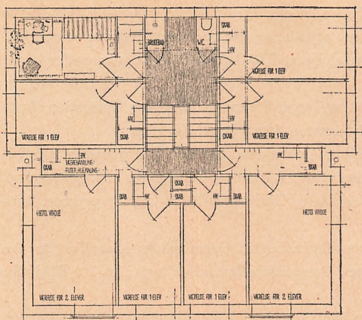
En Etage i et Elev-Kollegium med 8 Værelser til ialt 10 Beboere, samt Brusebad og W. C. Den nordlige og sydlige Del er forskudt ½ Etage i Forhold til hinanden.
