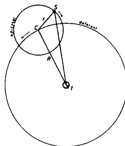
Apollonius' epicykelmodel
