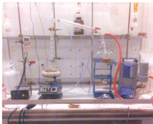
Vi fik desværre ingen billeder af eleverne i laboratoriet, men her ses destillationsopstillingen til oprensning af M-ester.
